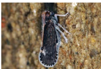
Cixiidae Indet. sp. 3
