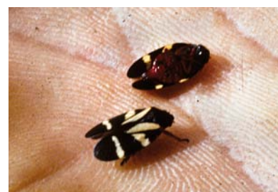
Cercopidae Indet. sp. 1
