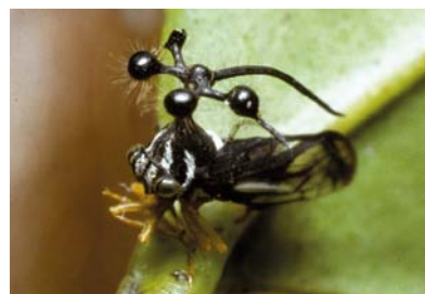
Membracidae Bocydium globulare
